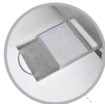
► Filtereinsatz im Grundboden des Generatorschranks integriert
